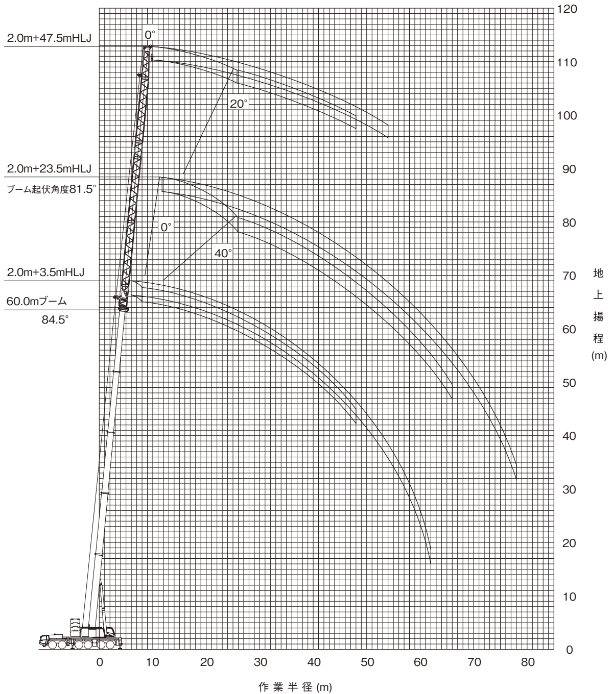
ブーム+油圧チルトジブ
