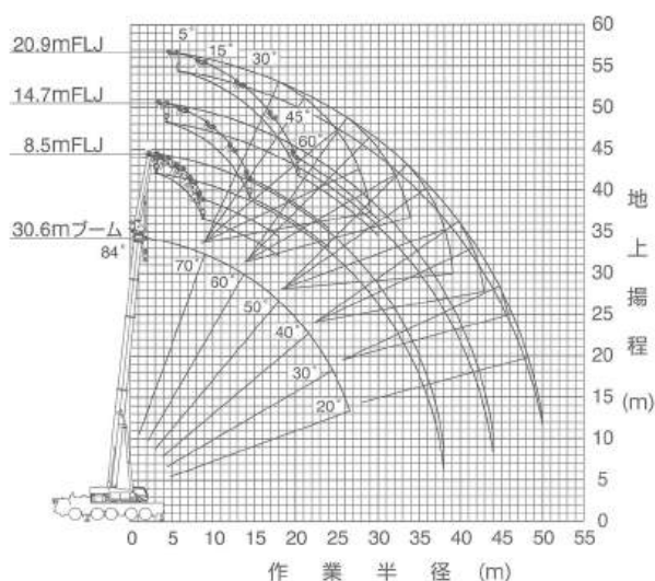
30.6mブーム+1.85m+フルオートラフィングジブ
