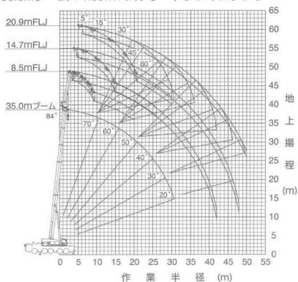
35.0mブーム+1.85m+フルオートラフィングジブ
